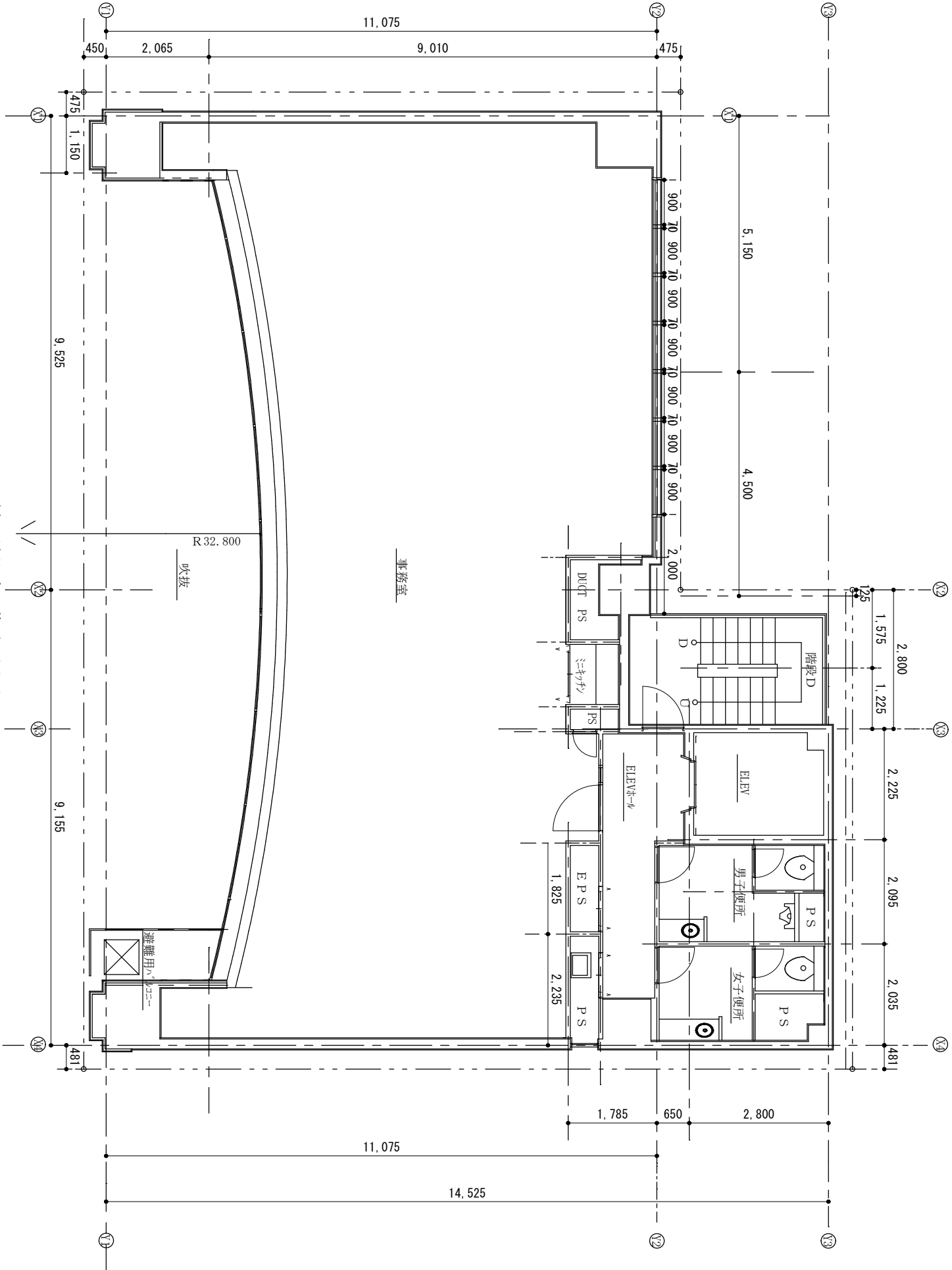
四ッ橋MT長谷ビル2階平面図1/100
