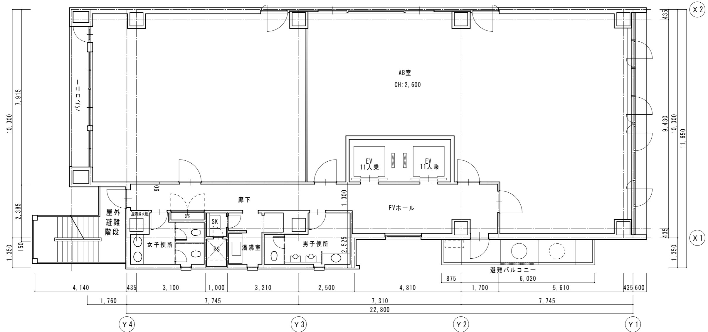
【8階平面図】
