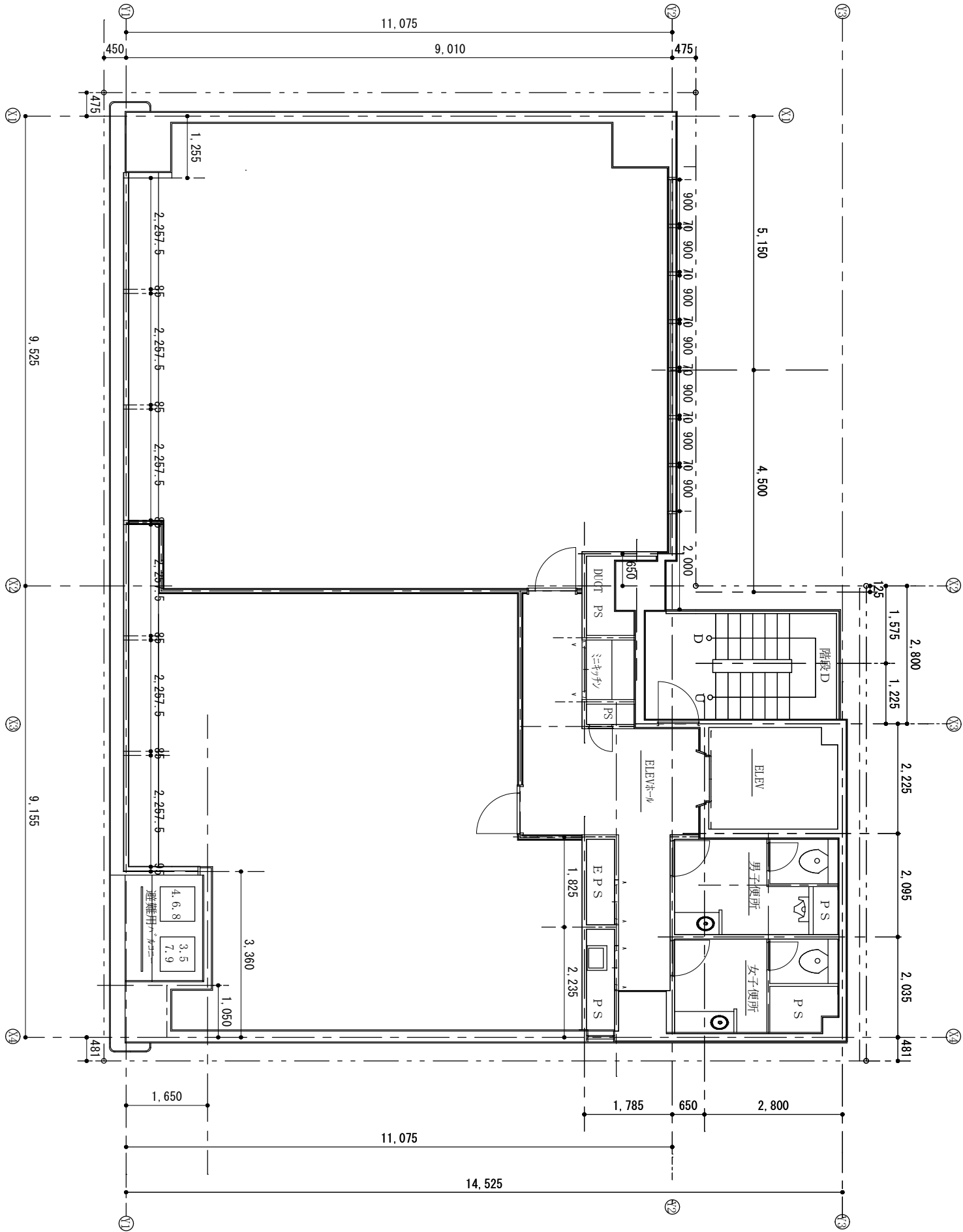
四ノ橋町長谷ビル3-9階平面図1/100
