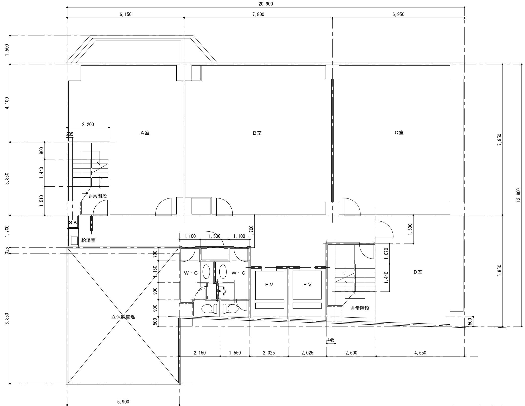
第11長谷ビル 基準階 平面図
